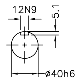
入力軸
