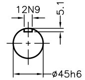
出力軸
